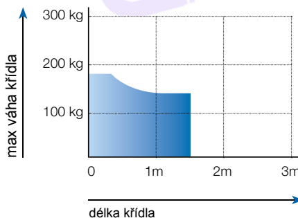
SCHEMA POUŽITÍ POSUVNÝCH RAMEN
