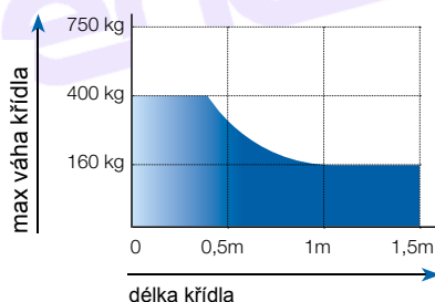
SCHEMA POUŽITÍ POSUVNÝCH RAMEN (reversibilní pohon)
