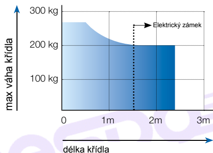
SCHEMA POUŽITÍ KLOUBOVÝCH RAMEN
